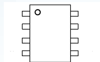
■ Simplified outline(ESOP-8)
